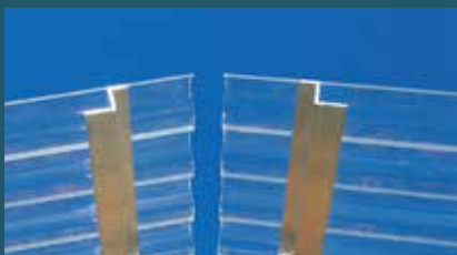
Firstabdeckung mit Abluftspalt
