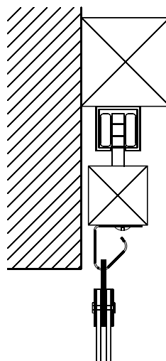
Montage als Schiebevorhang
