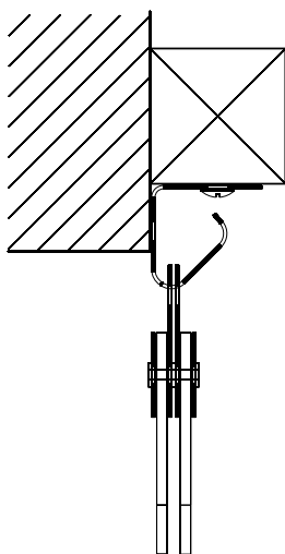
Montage vor Sturz
